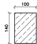
Section A-A
