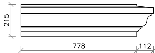
90° External Return - RH
