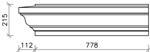
90° External Return - LH
