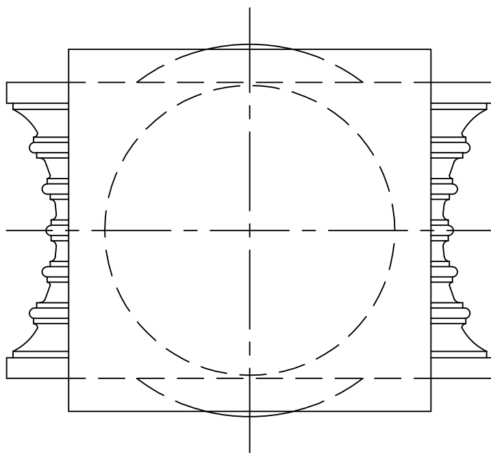
PLAN 1:5
