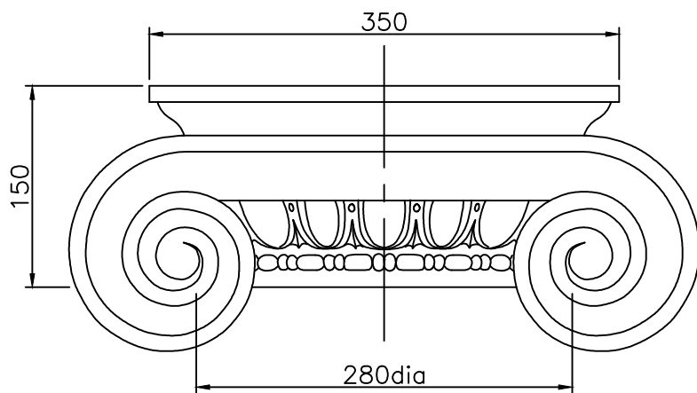
ELEVATION 1:5
