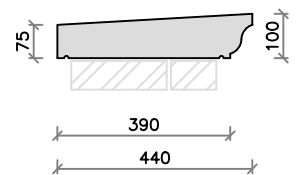
CS35 (46kg)
