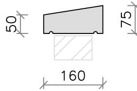
CS02 (13kg)
