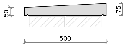
CS46 (42kg)
