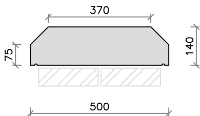
CS68 (83kg)
