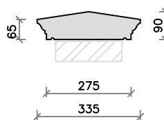
CS51 (30kg)
